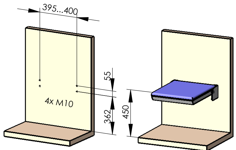
empfohlenes Lochbild
