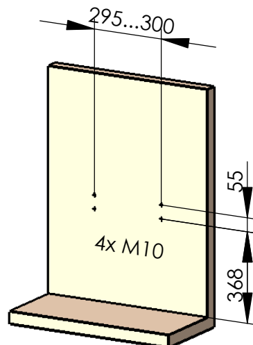
empfohlenes Lochbild
