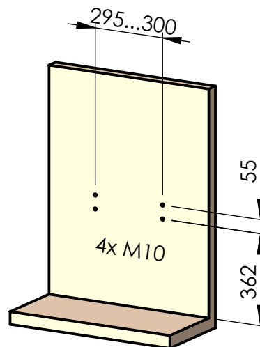
empfohlenes Lochbild
