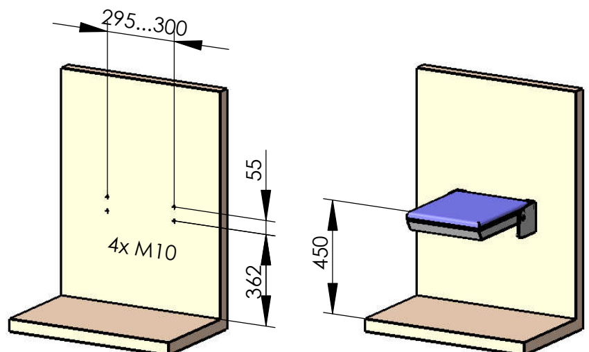
empfohlenes Lochbild
